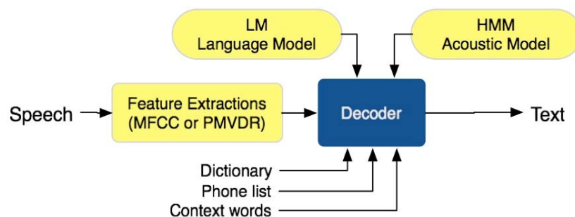
Figura 2: schema del sistema di riconoscimento di un file audio, comune ai software SONIC e SPHINX.
